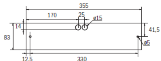
Bohrabstände KW Decke / Wand Drilling distances KW ceiling / wall
